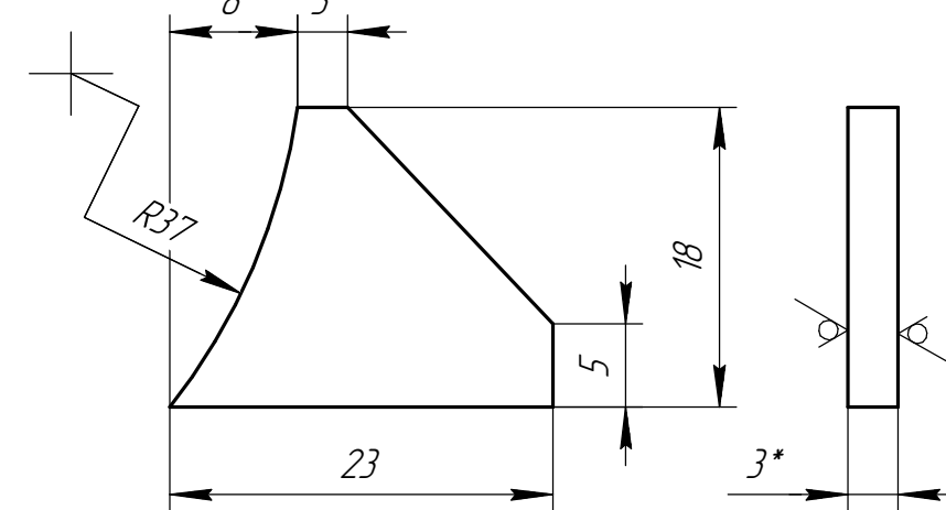
Дет. поз. 5 (2:1)
