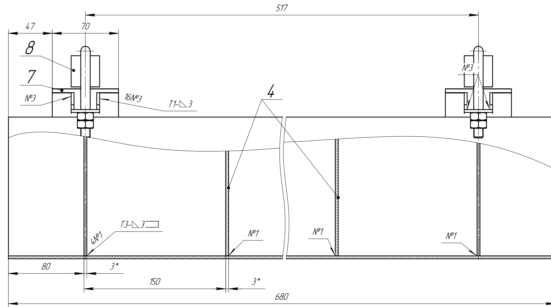
Дет. поз. 2 (1:1)
