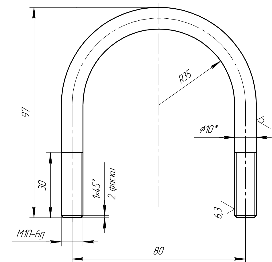
Дет. поз. 6 (1:1)
