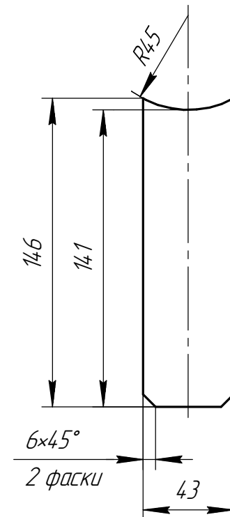
Дет. поз. 3 (1:2,5)
