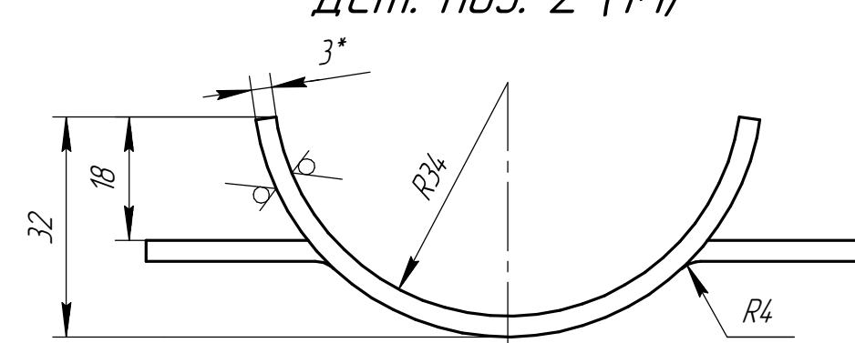
Дет. поз. 2 (1:1)
