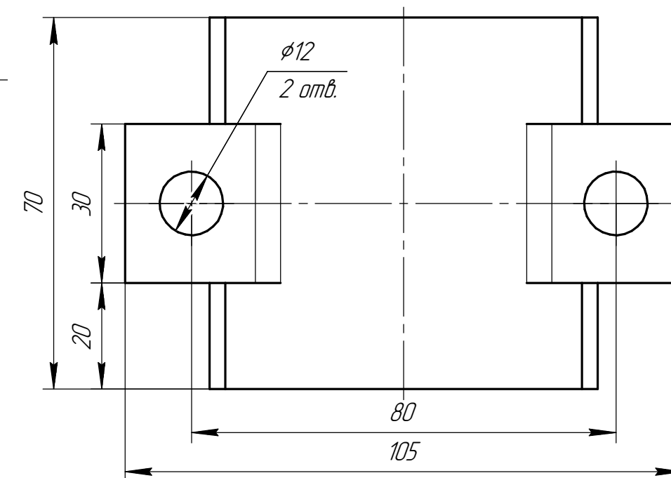
Дет. поз. 4 (1:2,5)
