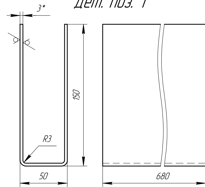
Дет. поз. 1
