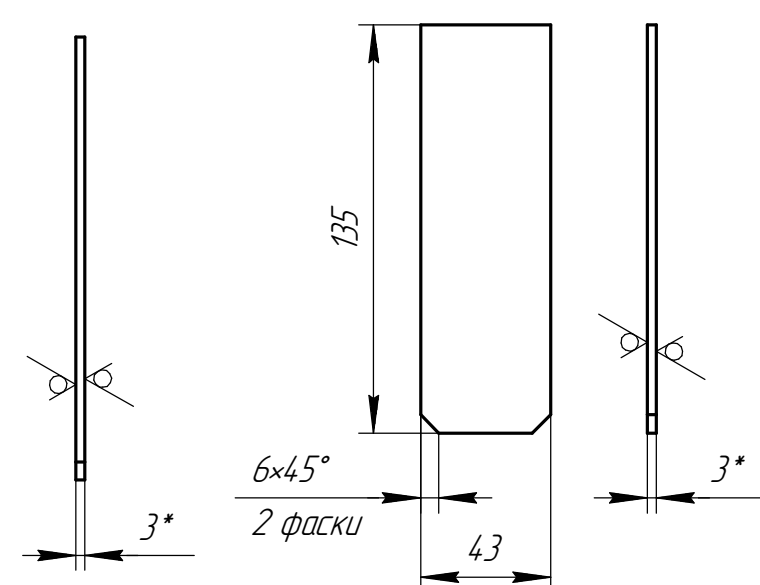
Дет. поз. 4 (1:2,5)
